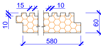
POPZECZNY PRZEKRÓJ PŁYTY POLISTYRENU EKSTRUDOWANEGO TECHNICOL CARBON DRENAŻ
