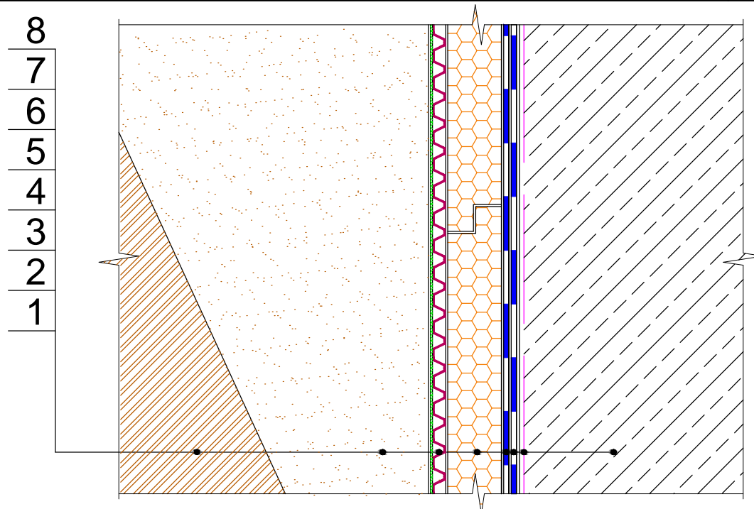
POPZECZNY PRZEKRÓJ PŁYTY POLISTYRENU EKSTRUDOWANEGO TECHNICOL CARBON DRENAŻ
